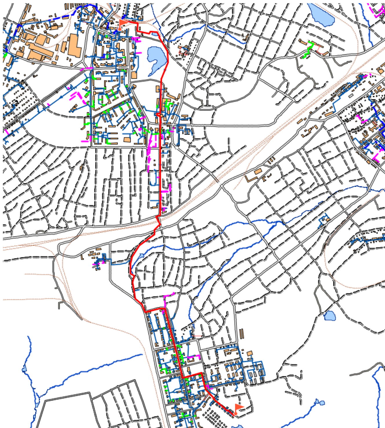
Рис. 5. Путь движения теплоносителя от ТЭЦ т/м V Южная до конечного потребителя
