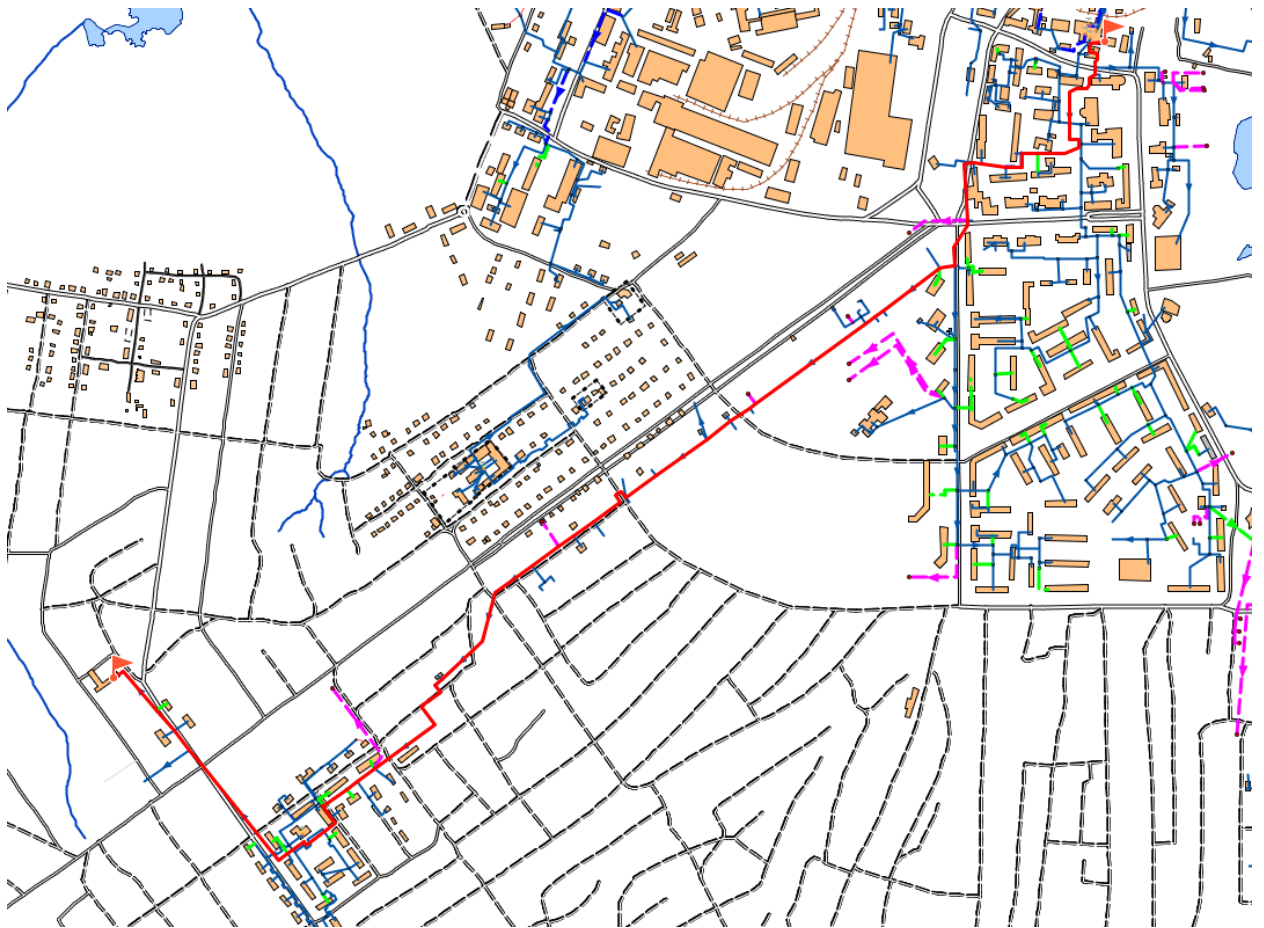
Рис. 2. Путь движения теплоносителя от ТЭЦ т/м II Желябова до конечного потребителя
