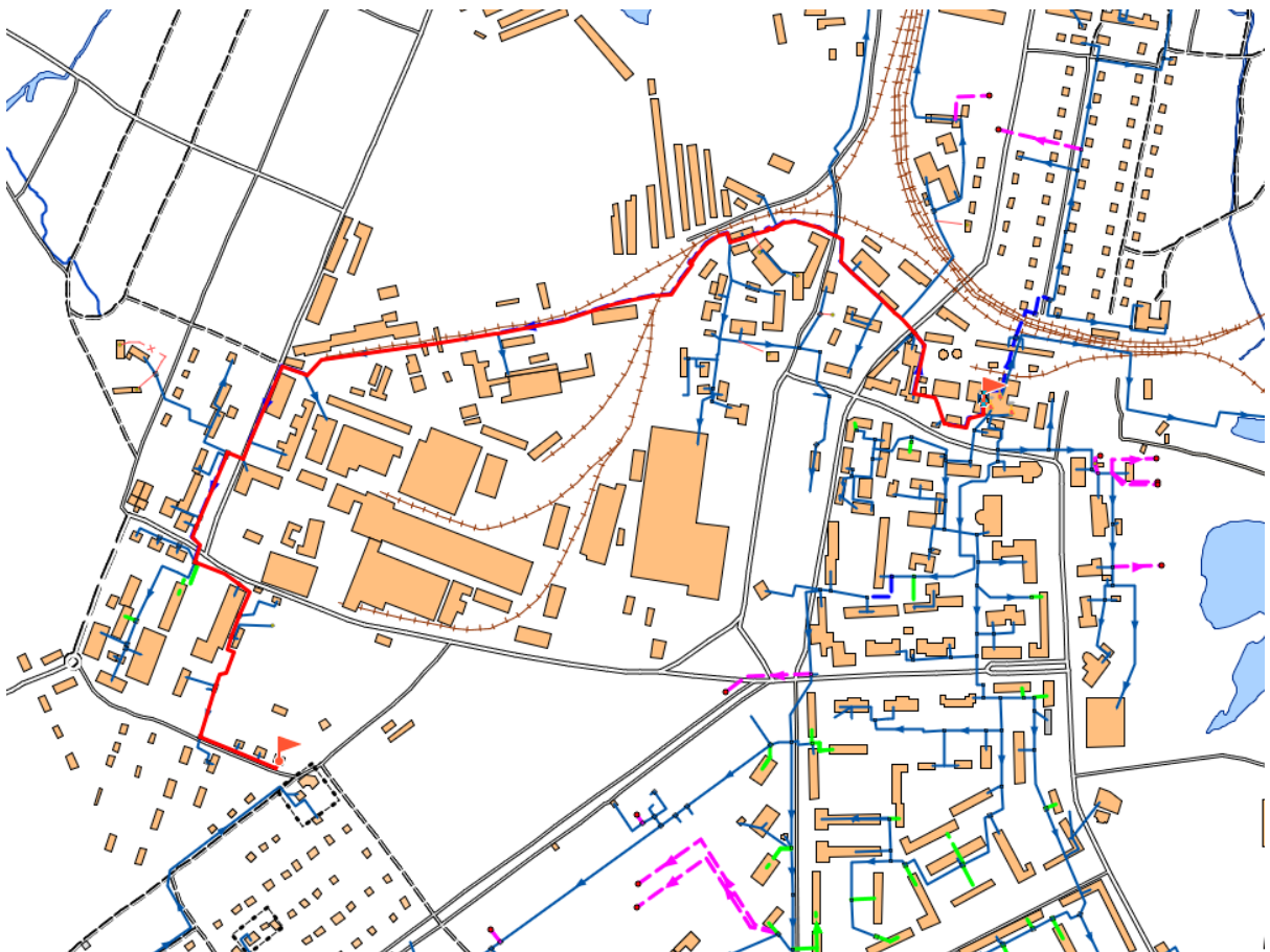
Рис. 3. Путь движения теплоносителя от ТЭЦ т/м III Машзавод до конечного потребителя
