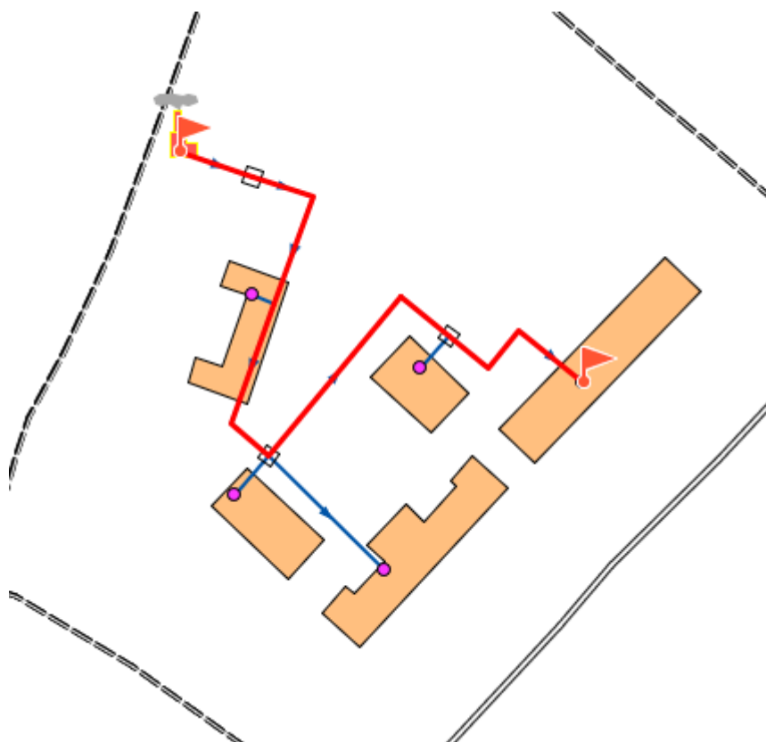
Рис. 9. Путь движения теплоносителя от котельной №5 до конечного потребителя
