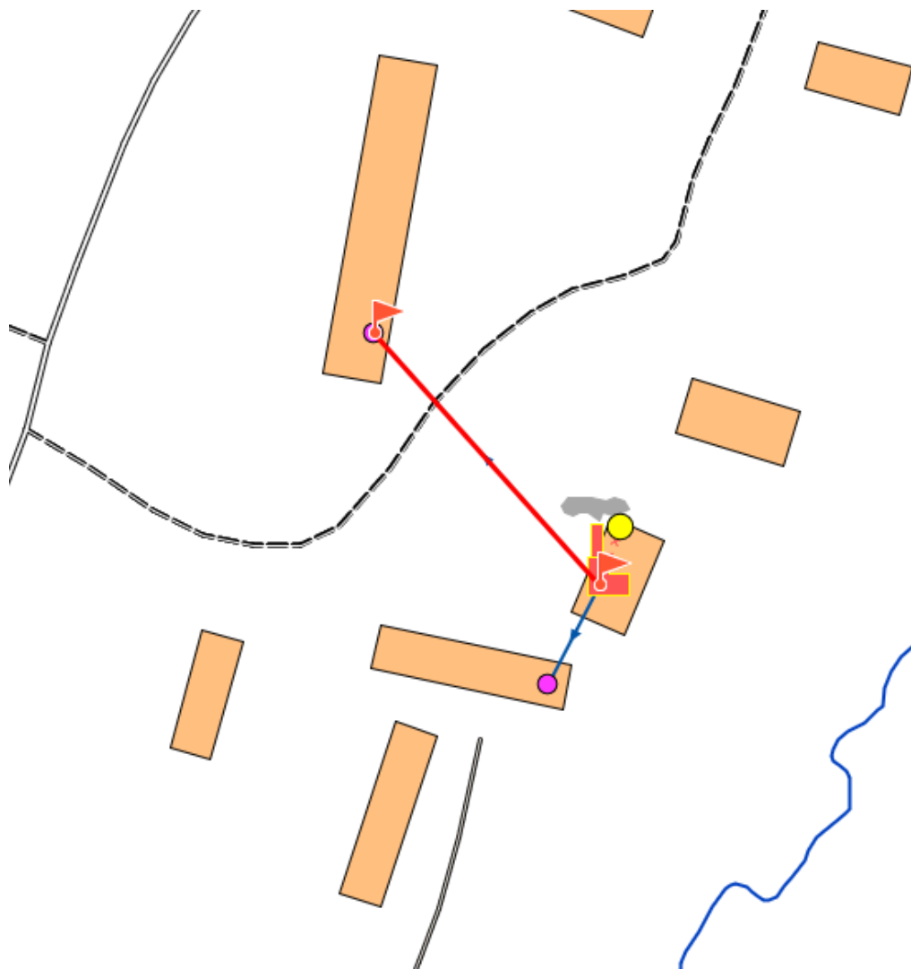
Рис. 25. Путь движения теплоносителя от котельной №27 до конечного потребителя
