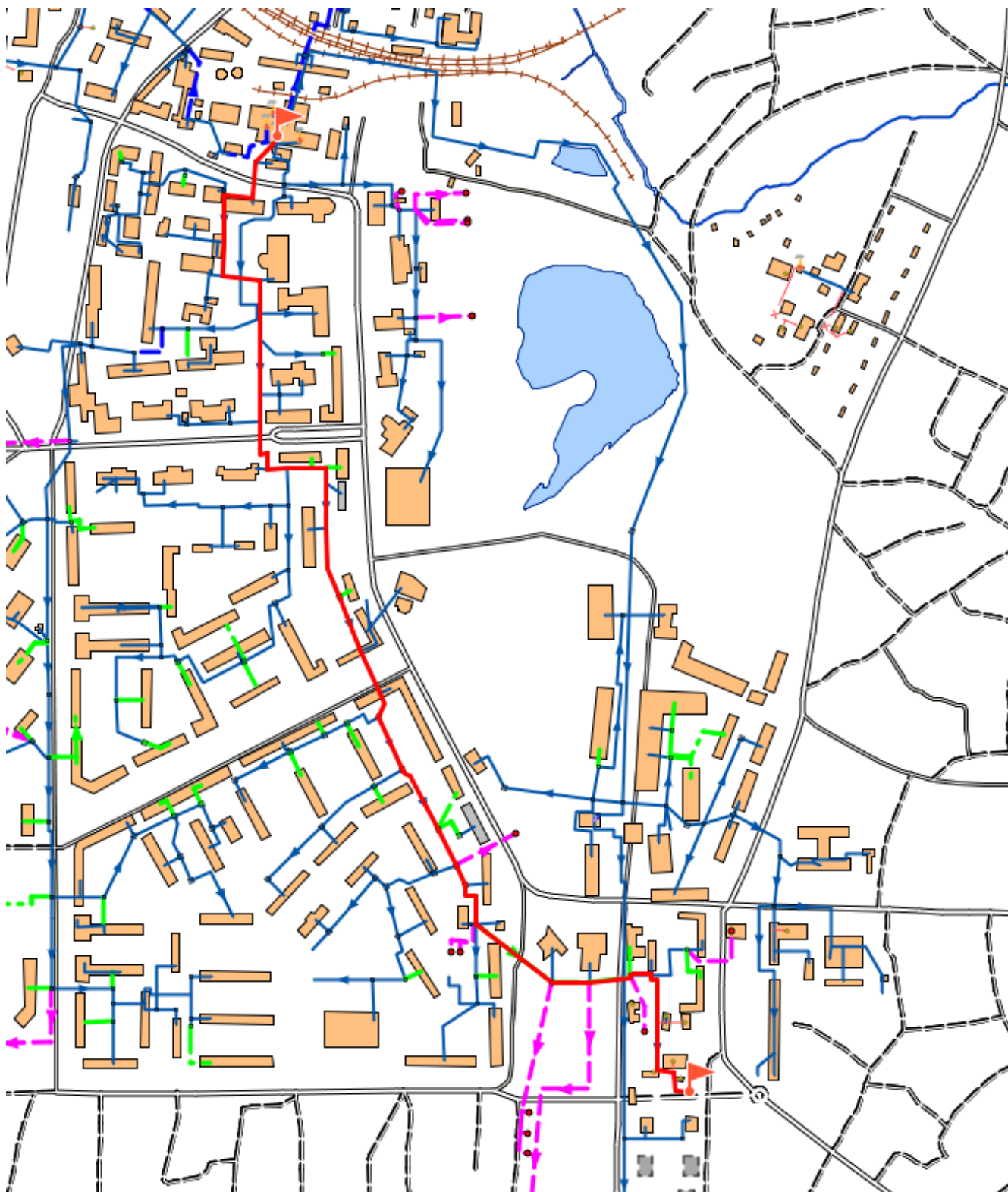
Рис. 1. Путь движения теплоносителя от ТЭЦ т/м I Город до конечного потребителя
