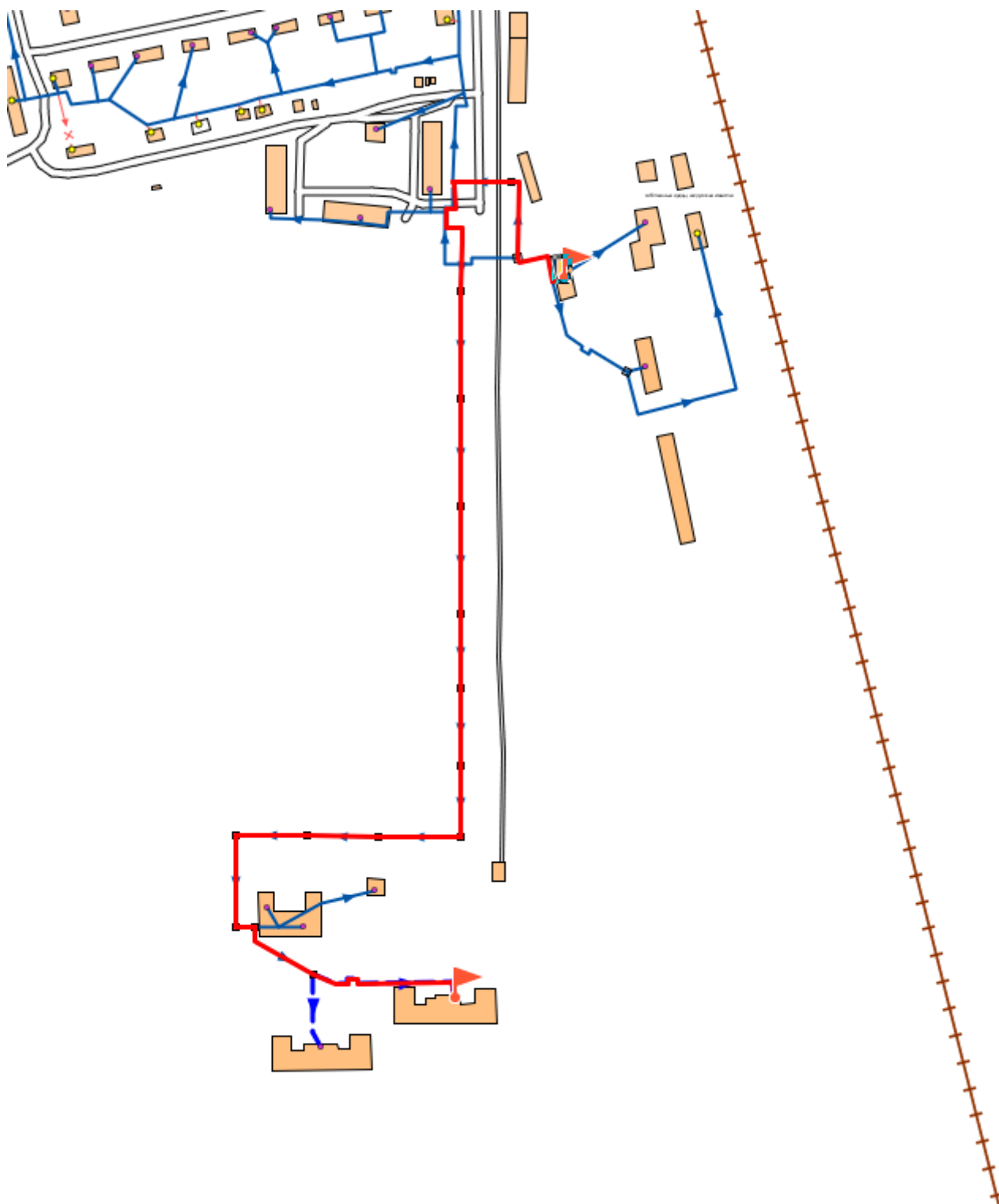
Рис. 20. Путь движения теплоносителя от котельной №20 до конечного потребителя
