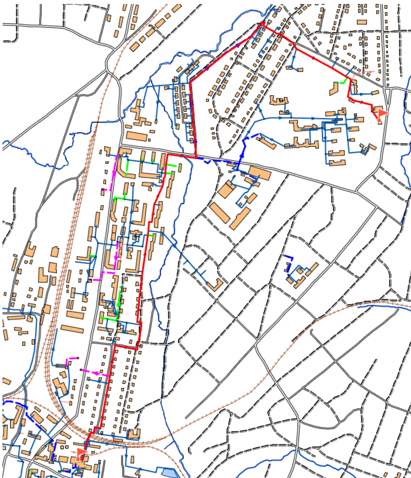
Рис. 4. Путь движения теплоносителя от ТЭЦ т/м IV Совхоз до конечного потребителя
