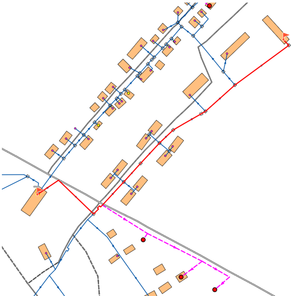
Рис. 21. Путь движения теплоносителя от котельной №23 до конечного потребителя
