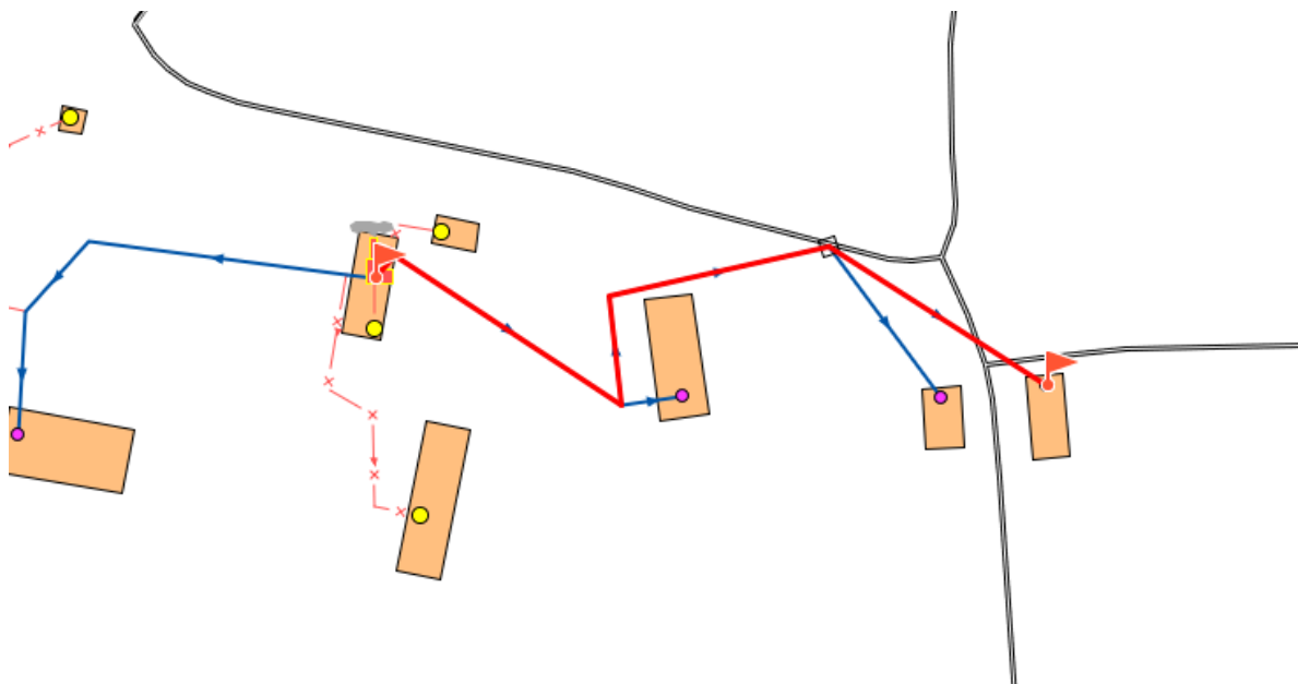
Рис. 26. Путь движения теплоносителя от котельной №29 до конечного потребителя
