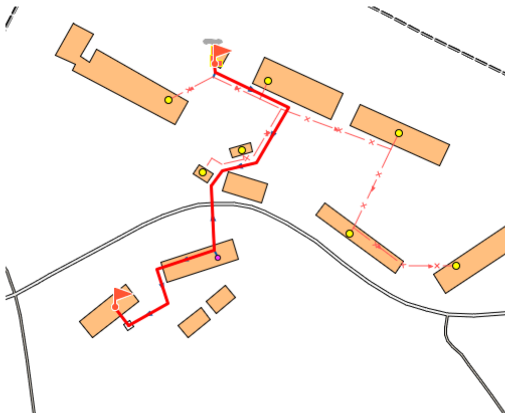
Рис. 19. Путь движения теплоносителя от котельной №19 до конечного потребителя
