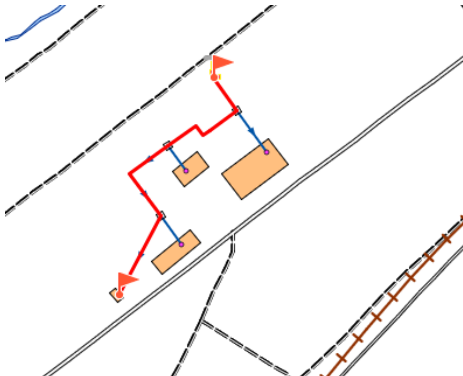
Рис. 13. Путь движения теплоносителя от котельной №9 до конечного потребителя
